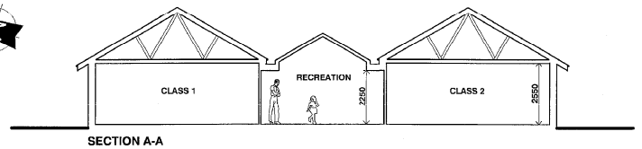
SECTION A-A
